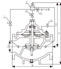
1、小球阀 2、导阀 3、小球阀 4、小球阀 5、针形阀
