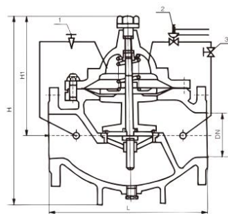
1、针型阀 2、导阀 3、球阀
